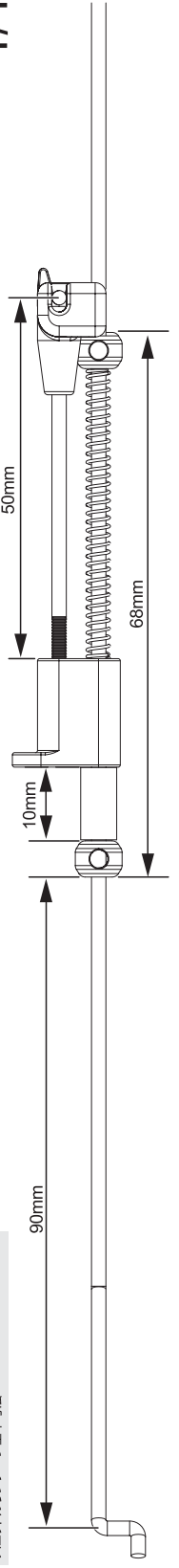
STANDARD THROTTLE LINKAGE DIMENSION スロットルリンクアームの基本寸法
